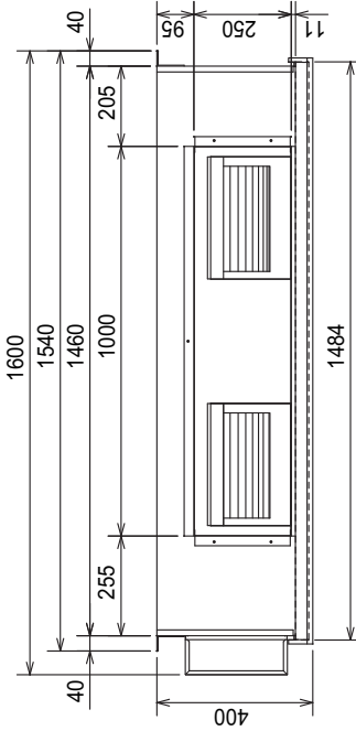
Вид сверху
