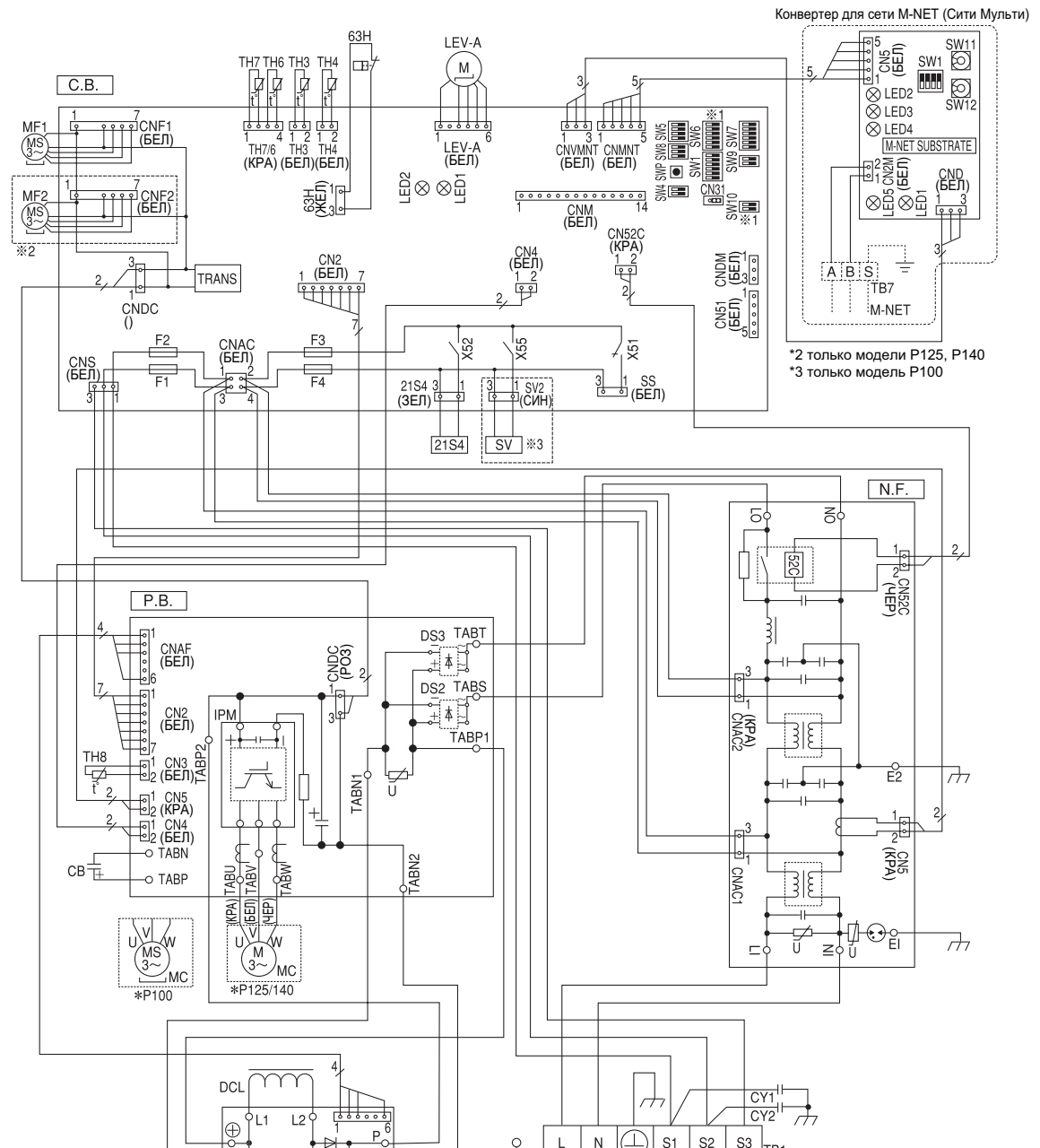
Конвертер для сети M-NET (Сити Мульти)
