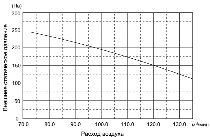
PEA-RP400GA
