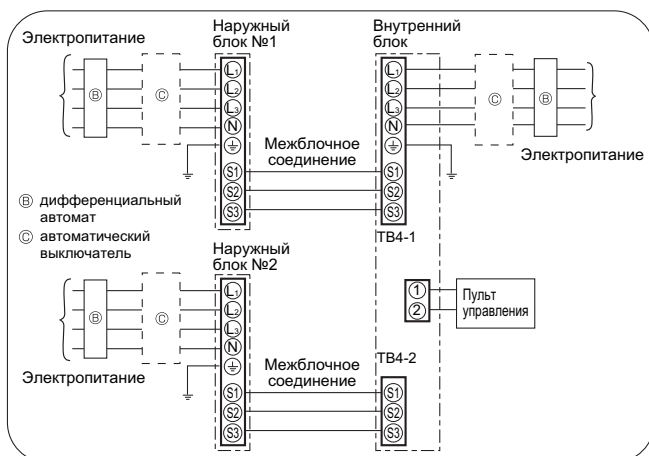
Система 2:1 (внутренние блоки PEА-RP400/500GA)
