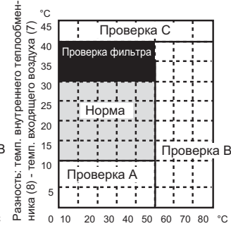
Режим обогрева
