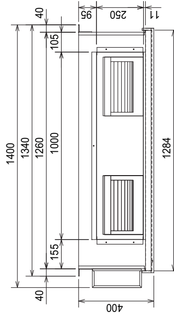
Вид сверху
