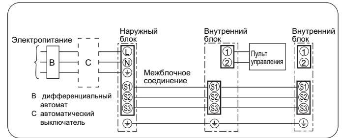
• Синхронная двойная система (система 1:2)
