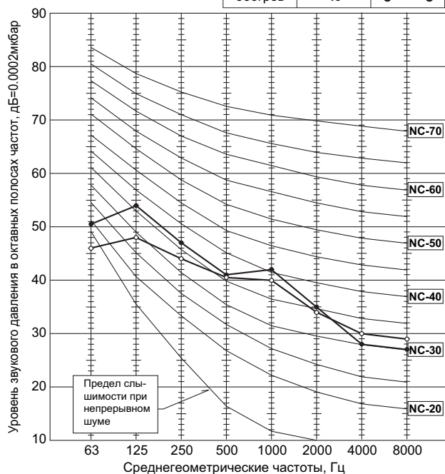
PUHZ-RP35VHA2 PUHZ-RP50VHA2
