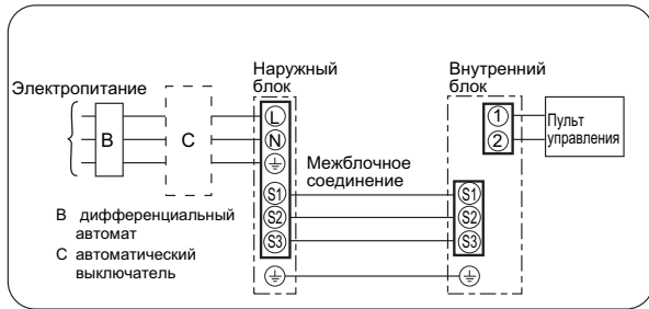
Система 1:1
