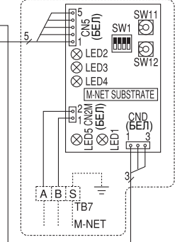
Конвертер для сети M-NET (Сити Мульти)
