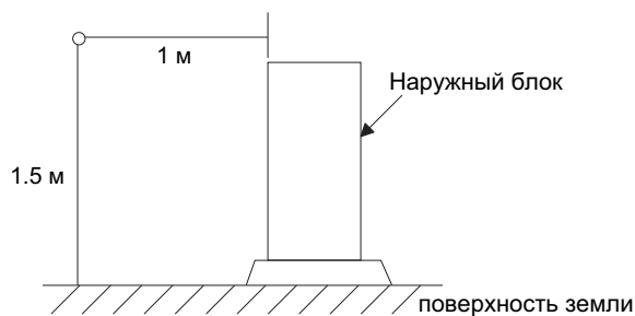
PUHZ-RP60VHA2 PUHZ-RP71VHA2
