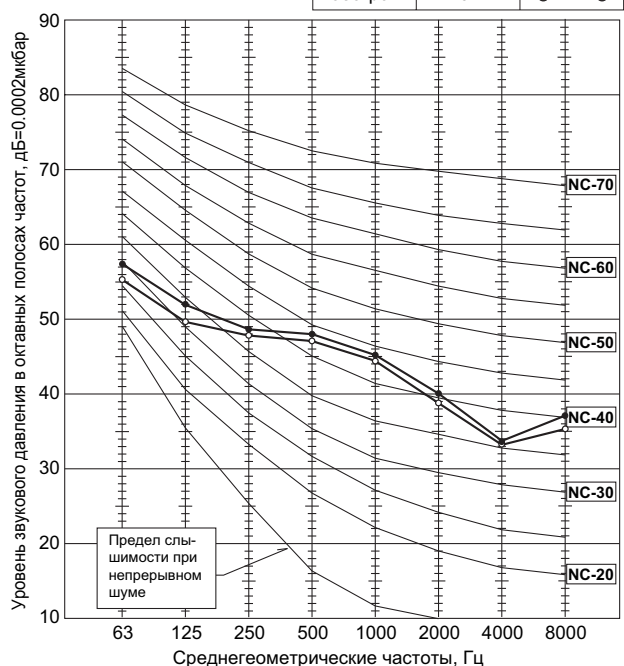
PUHZ-RP100VHA2 PUHZ-RP100YHA2
