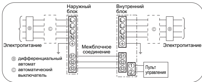
Система 1:1 (внутренние блоки PEА-RP200/250GA)
