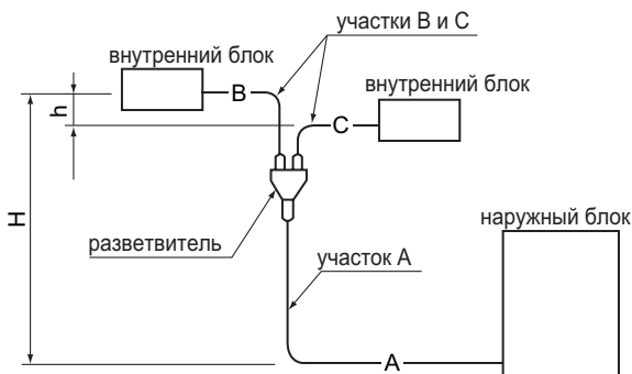
Система 1:2
