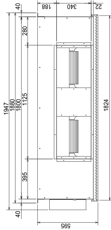
Вид спереди
