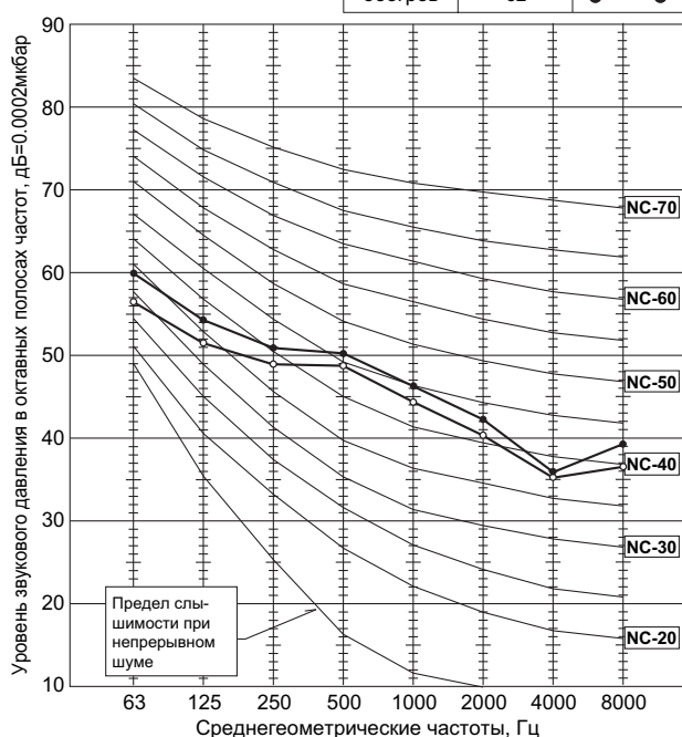
PUHZ-RP125/140VHA2 PUHZ-RP125/140YHA2
