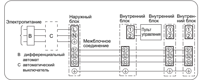
• Синхронная тройная система (система 1:3)
