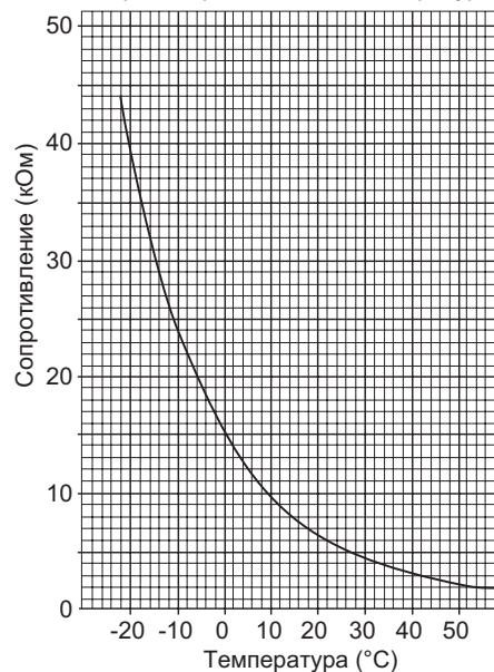
Термистор для низких температур
