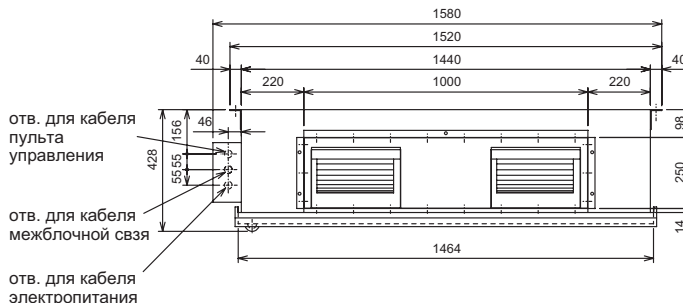
Вид спереди
