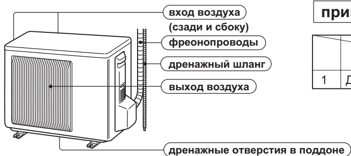
наружный блок
