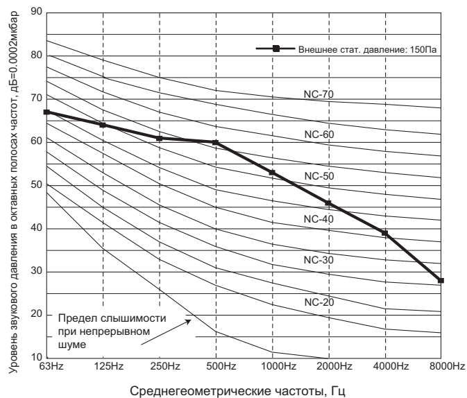
PEH-P500MYA
