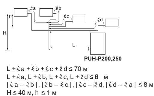
(4) Система «1 : 4»
