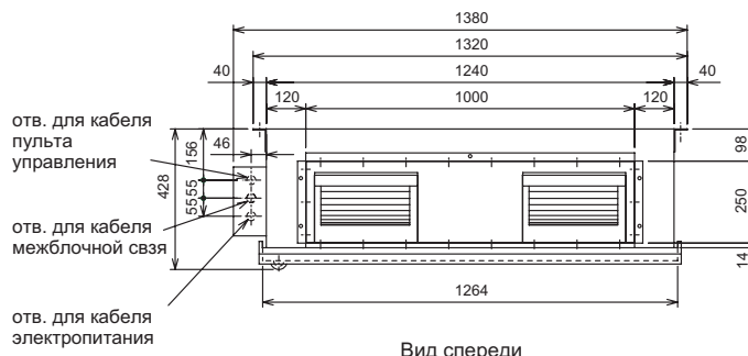
Вид спереди
