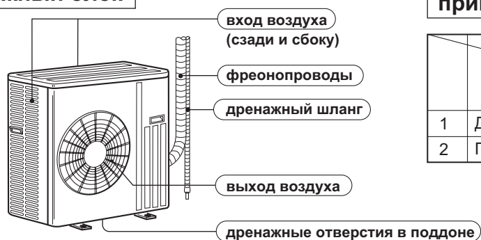
наружный блок
