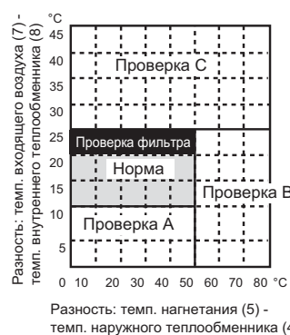
Режим охлаждения
