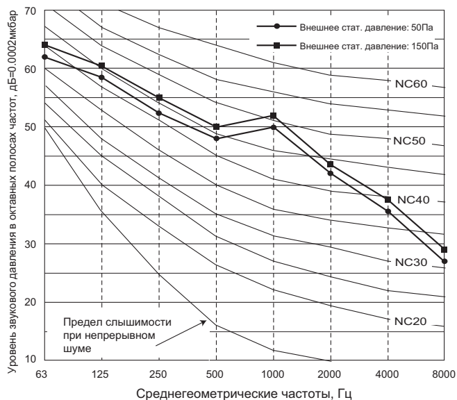
РЕН-RP250MYA
