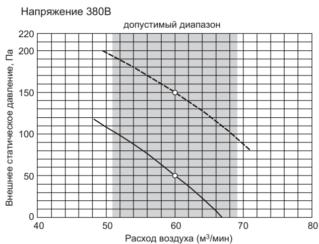
РЕН-RP200MYA
