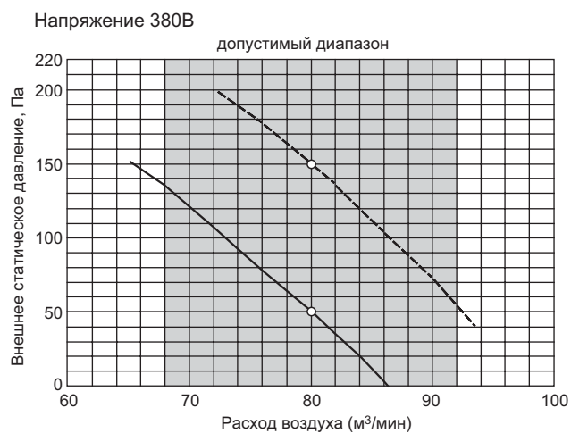
РЕН-RP250MYA
