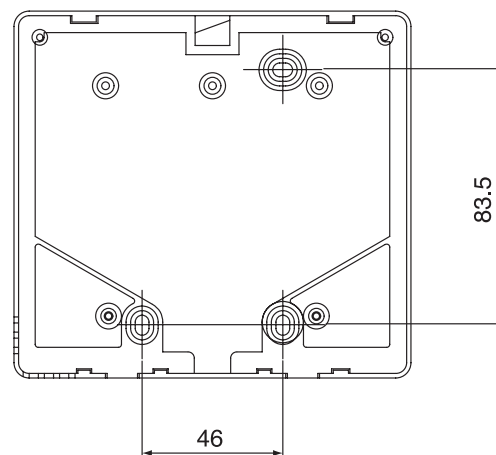
Вид сзади
