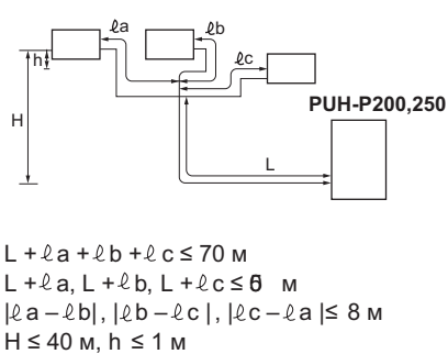
(3) Система «1 : 3»
