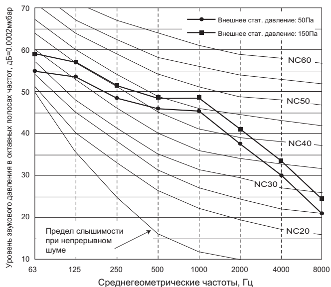
РЕН-RP200MYA
