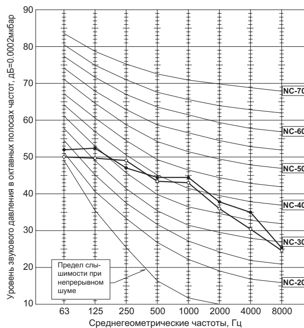
PUHZ-RP60VHA2 PUHZ-RP71VHA2
